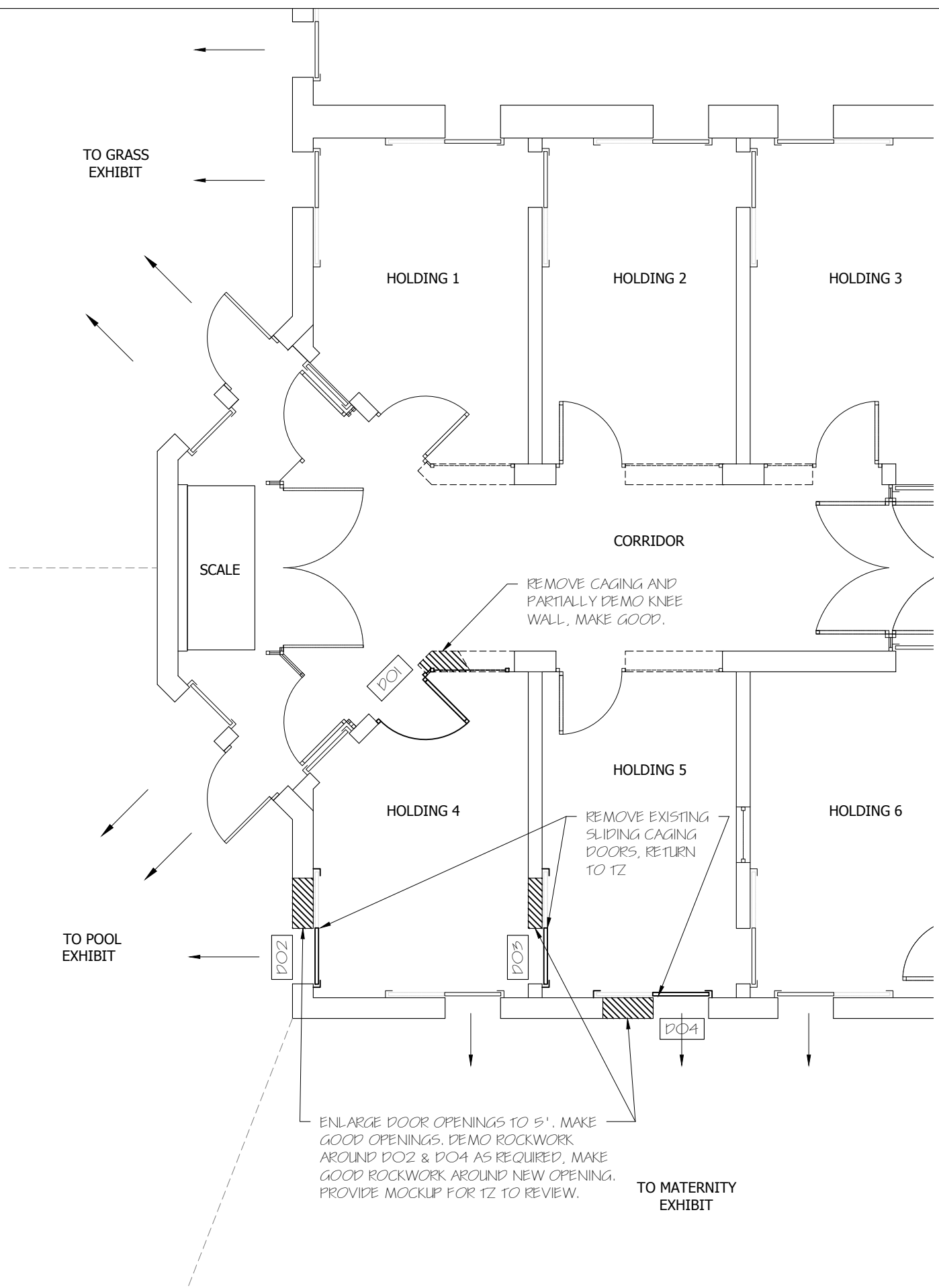
1 DEMO FLOOR PLAN Scale: 1:100
